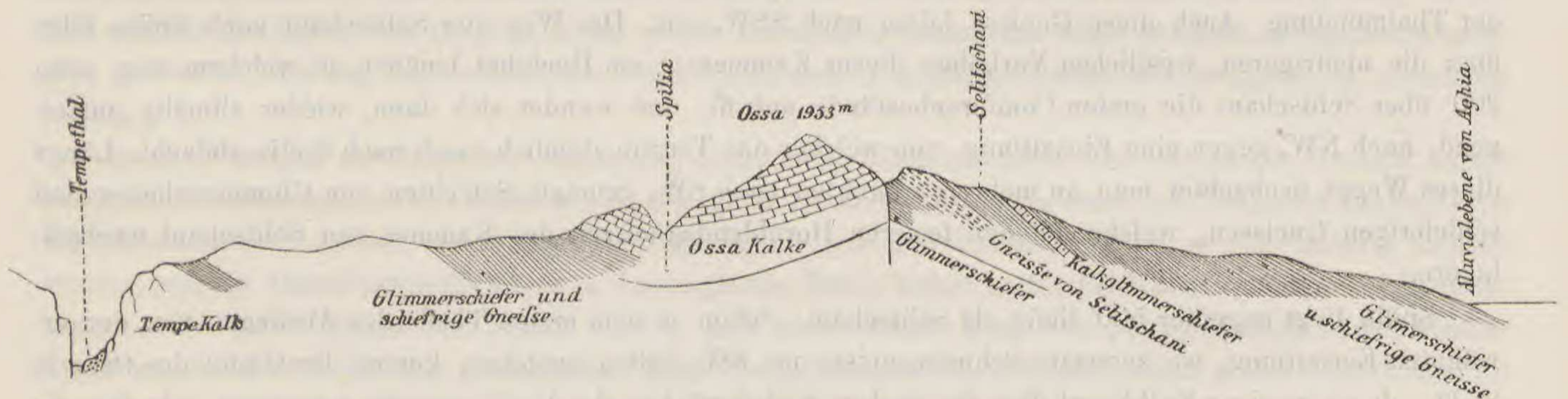
Fig. 4. Idealer Durchschnitt durch den Gebirgsstock des Ossa.
